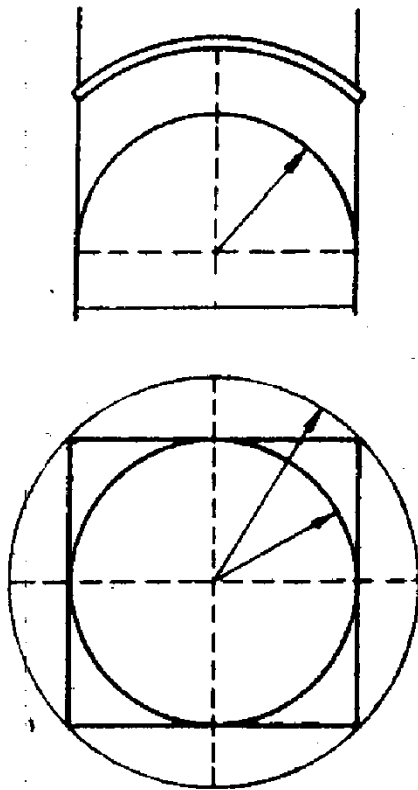
Rys. 5-5. Sklepienie żagłowe
