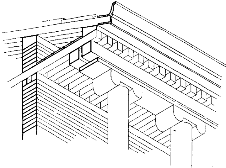
173. Porządek joński, drewniany pierwowzór
