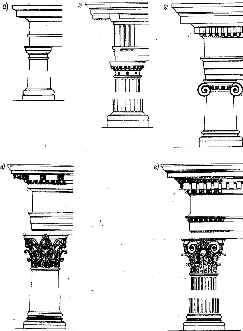
Rys. 5-8. Porządki rzymskie: a) toskański, b) rz.-dorycki, c) rz.-joński, d) rz.-koryncki, e) kompozytowy
