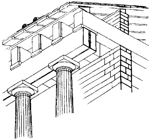
171. Porządek dorycki, drewniany pierwowzór
