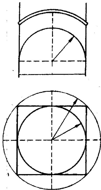
Rys. 5-5. Sklepienie żaglowe
